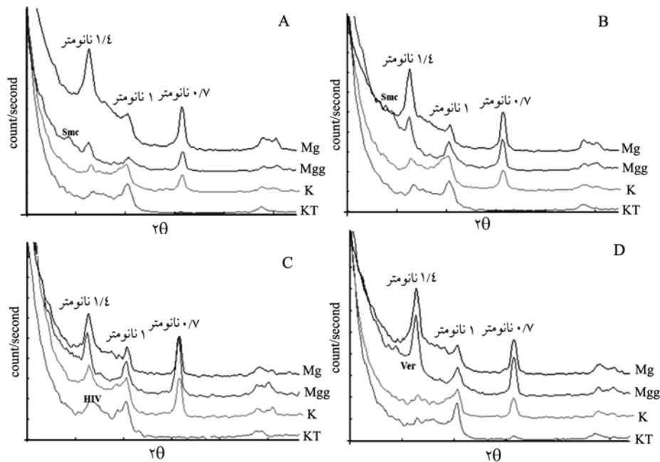
شکل ۲- دیفراکتوگرام برخی نمونه‌های مورد مطالعه، A: افق Btg_2 خاک رخ ۳، B: افق Btg_2 خاک رخ ۴، C: افق Btg_2 خاک رخ ۶، D: افق Btg_1 خاک رخ ۷.
