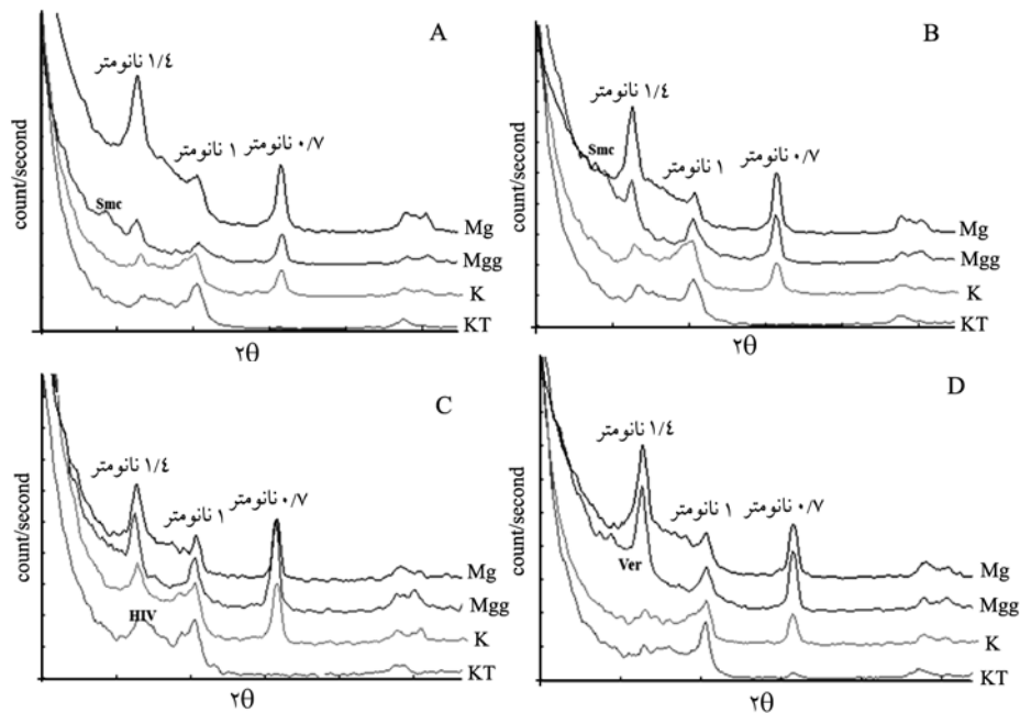
شکل ۲- دیفراکتوگرام برخی نمونه‌های مورد مطالعه، A: افق Bg_2 خاک رخ ۳، B: افق Bg_2 خاک رخ ۴، C: افق Bg_2 خاک رخ ۶، D: افق Btg_1 خاک رخ ۷.
