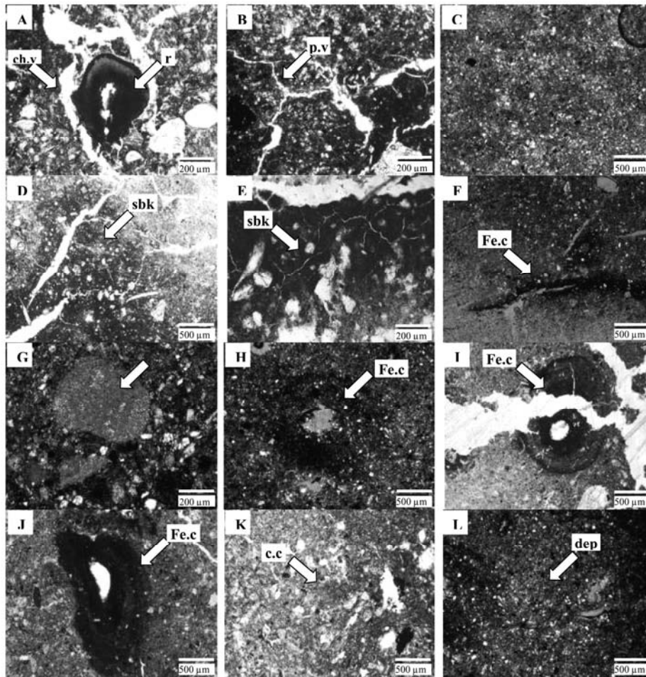
شکل ۳- تصاویر میکروسکوپ پلاریزان- A (Apg خاک رخ ۲): بقایای در حال پوسیدگی ریشه (r) در کنار حفرات کانالی (ch.v)، B (Apg خاک رخ ۳): حفرات کانالی و صفحه‌ای (p.v)، C (Bg ۳ خاک رخ ۴): خاک‌دانه‌های توده‌ای و بدون حفرات مشخص، D (Btg ۱ خاک رخ ۴): خاک‌دانه مکعبی با تفکیک متوسط تا ضعیف (sbk)، E (Bg ۲ خاک رخ ۶): خاک‌دانه مکعبی با تفکیک متوسط تا خوب، F (Btg ۱ خاک رخ ۴): پوشش آهن در امتداد ریشه پوسیده (Fe.c)، G (Bg ۱ خاک رخ ۱): پوشش زیرسطحی آهن در اطراف ندول کربناته، H (۳Bg ۲ خاک رخ ۴): پوشش زیرسطحی و در امتداد سطح آهن (Quasi-coating) در اطراف حفرات، I (Bg ۱ خاک رخ ۶): پوشش زیرسطحی و در امتداد سطح آهن در اطراف حفرات، J (Bg ۱ خاک رخ ۶): پوشش کفه نازک آهن (Micropan)، K (Btg ۱ خاک رخ ۷): پوسته رسی (c.c)، L (۳Bg ۲ خاک رخ ۴): مناطق تخلیه شده از آهن در اطراف تجمعات (dep).
