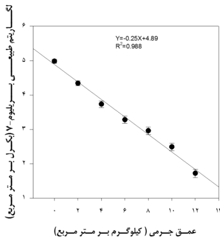
شکل ۵- رگرسیون خطی بین لگاریتم طبیعی فعالیت بریلیم-۷ \ln[A(x)] و عمق جرمی (x) .
