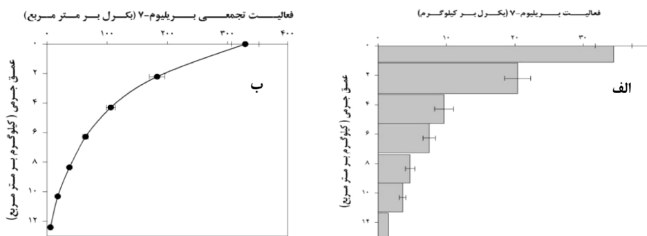
شکل ۴- الف) توزیع عمقی فعالیت جرمی و ب) فعالیت تجمعی برلیوم-۷ در واحد سطح در پروفیل مرجع.
