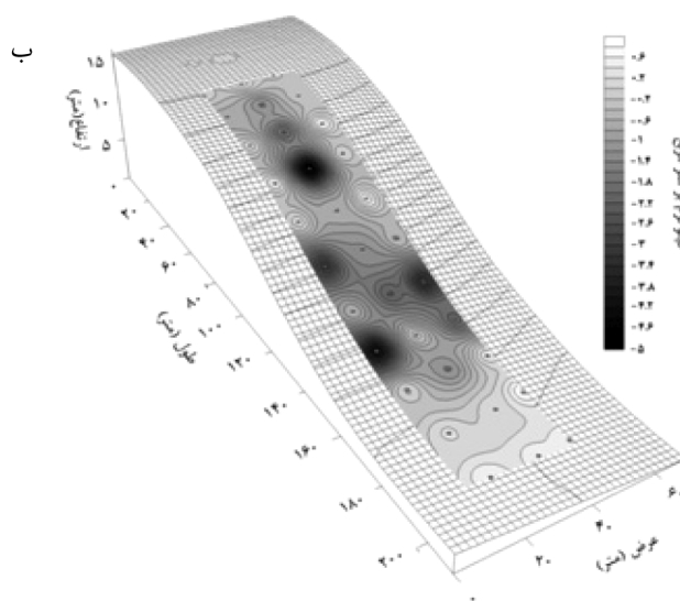
شکل ۶- الف) توزیع موجودی یرلیوم-۷ (بکرل بر مترمربع) و ب) نقشه توزیع مجدد خاک (کیلوگرم بر مترمربع) (مقادیر منفی نشان‌دهنده فرسایش و مقادیر مثبت رسوب می‌باشند) با استفاده از روش میانگین وزنی عکس فاصله در دامنه شیب مورد مطالعه و موقعیت نقاط نمونه‌برداری.
