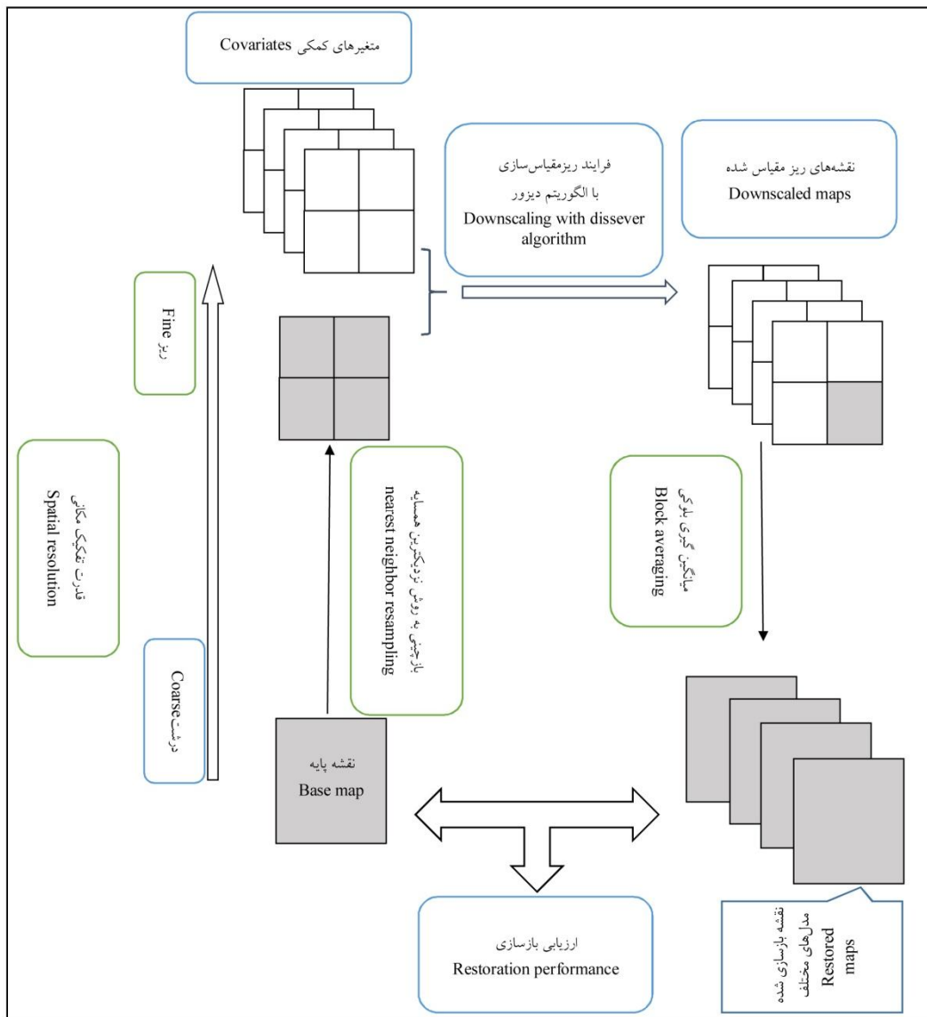
شکل ۲- فلوچارت مراحل مختلف ریزمقیاس سازی با الگوریتم دیزور.
