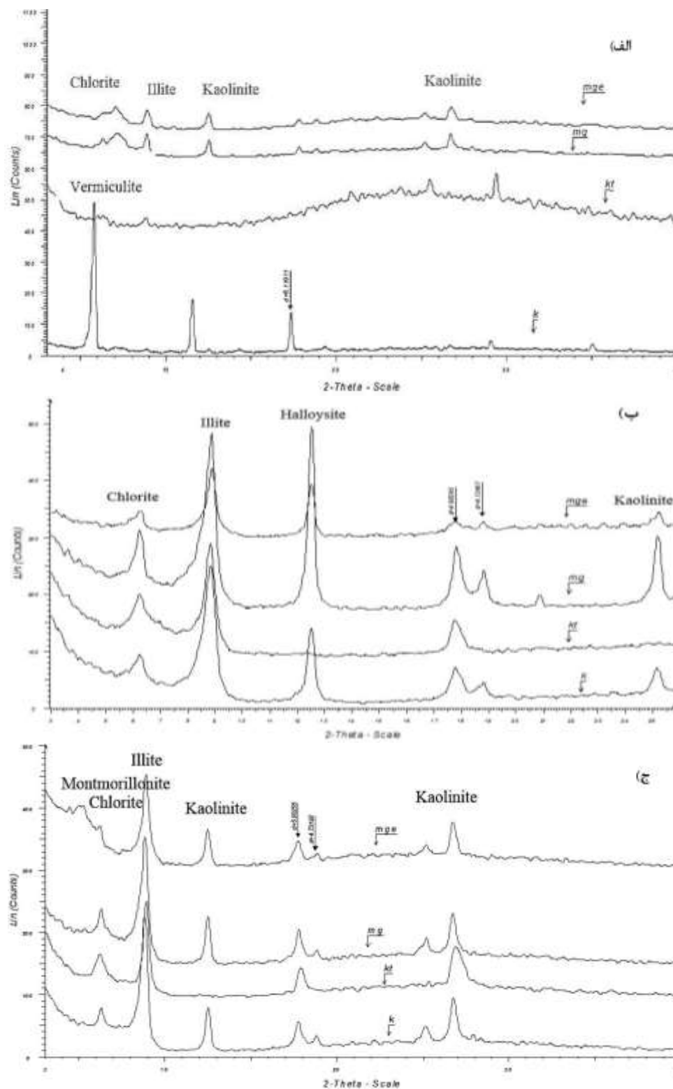
شکل ۵- پراش‌نگارهای کانی‌شناسی رس در افق 2C خاکرخ ۲ (الف)، افق Btnz1 خاکرخ ۳ (ب) و افق Bkzrn خاکرخ ۷ (ج). k: اشباع با پتاسیم، kt: اشباع با پتاسیم و تیمار حرارت ۵۵۰ درجه سلسیوس. mg: تیمار اشباع با منیزیم، mge: اشباع با منیزیم و تیمار اتیلن گلیکول.
