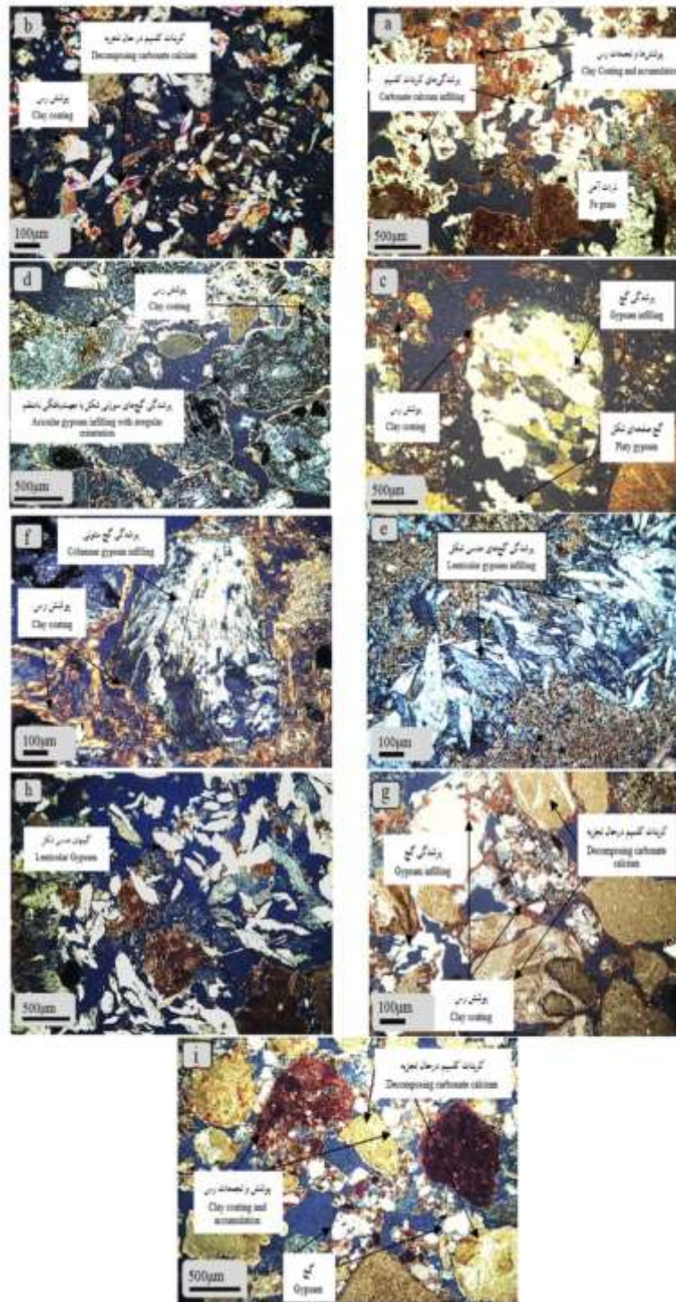
شکل ۲- تصاویر میکروسکوپی مقاطع نازک در حالت نور متقاطع (XPL). a: خاکرخ ۲ در عمق ۹۰-۱۳۵ سانتی‌متر (2Btkn)، b: خاکرخ ۲ در عمق ۲۵-۵۵ سانتی‌متر (Btkyz)، c: خاکرخ ۳ در عمق ۱۰-۴۰ سانتی‌متر (Bkzn)، d: خاکرخ ۷ در عمق ۴۵-۸۵ سانتی‌متر (Bkn)، e: خاکرخ ۷ در عمق ۱۰-۴۵ سانتی‌متر (Bkyzn)، f: خاکرخ ۶ در عمق ۳۵-۶۵ سانتی‌متر (Bw)، g: خاکرخ ۵ در عمق ۶۰-۱۱۵ سانتی‌متر (Bky2)، h: خاکرخ ۱ در عمق ۳۰-۴۵ سانتی‌متر (Bk)، i: خاکرخ ۴ در عمق ۴۰-۷۰ سانتی‌متر (Btkn).
