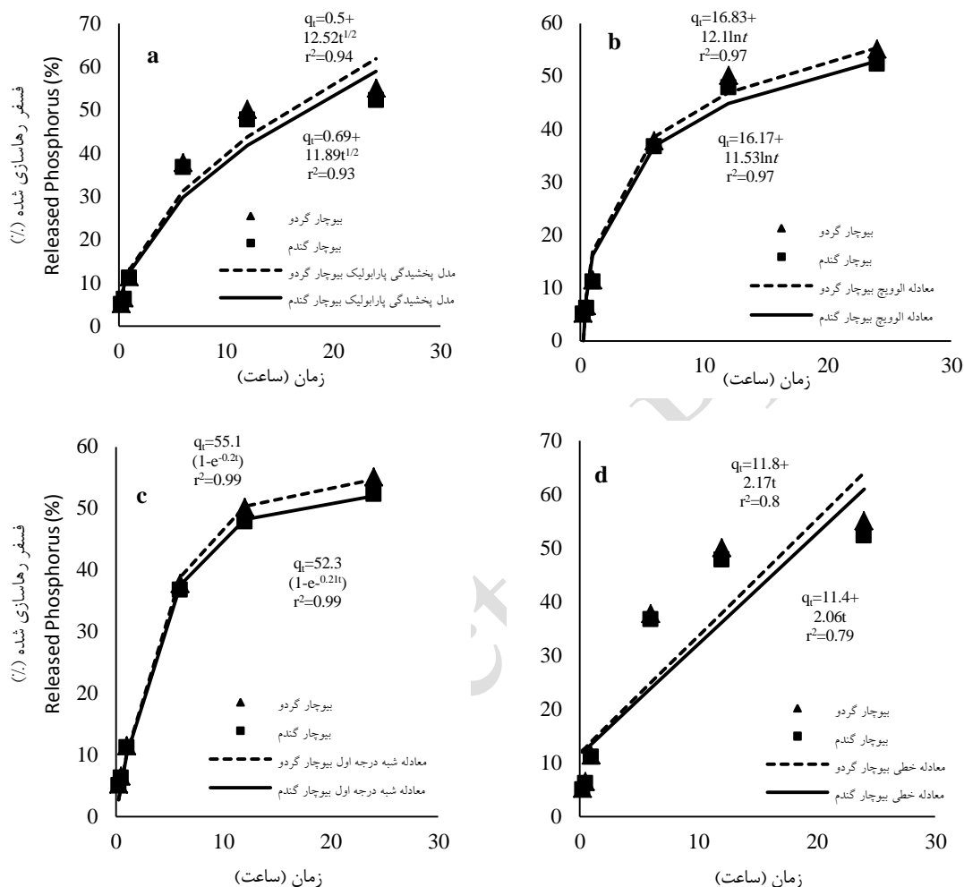
شکل ۱۱- مدل پنخشیدگی پارابولیک (a)، معادله الویچ (b)، معادله شبه درجه اول غیر خطی (c) و معادله خطی (d) برازش شده برای بیوجار پوست گردو و بیوجار کلش گندم در کمپوزیت‌های فسفردار پایه بیوجار-اکسید/هیدروکسید آهن در زمان صفر تا ۲۴ ساعت.
