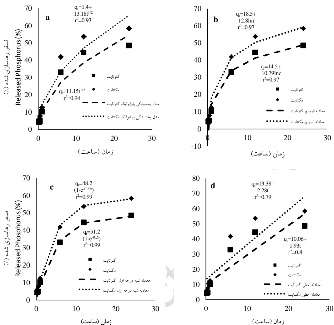
شکل ۱۲- مدل پخشیدگی پارابولیک (a)، معادله الوویچ (b)، معادله شبه درجه اول غیر خطی (c) و معادله خطی (d) برازش شده برای گئوتایت و مگنتایت در کمپوزیت‌های فسفردار پایه بیوجار-اکسید/هیدروکسید آهن در زمان صفر تا ۲۴ ساعت.
