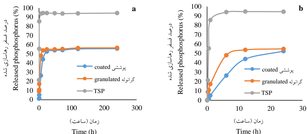
شکل ۹- مقایسه میانگین اثر نوع کود (پوشش داده شده، گرانوله شده و سوپرفسفات تریپل (TSP)) بر درصد رهاسازی فسفر از کمپوزیت‌های کودی فسفردار پایه بیوجار-اکسید/هیدروکسید آهن در طی زمان صفر تا ۲۴۰ ساعت (a) و زمان صفر تا ۲۴ ساعت (b).
