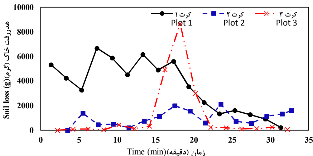
شکل ۲- تغییرات زمانی تولید رواناب (بالا) و هدررفت خاک (پایین) در کرت‌های آزمایشی مطالعاتی واجد فرسایش شیاری.
